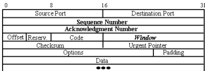
Fig. 12. TCP segment format
